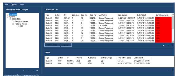
Figure 12: SAM Module
